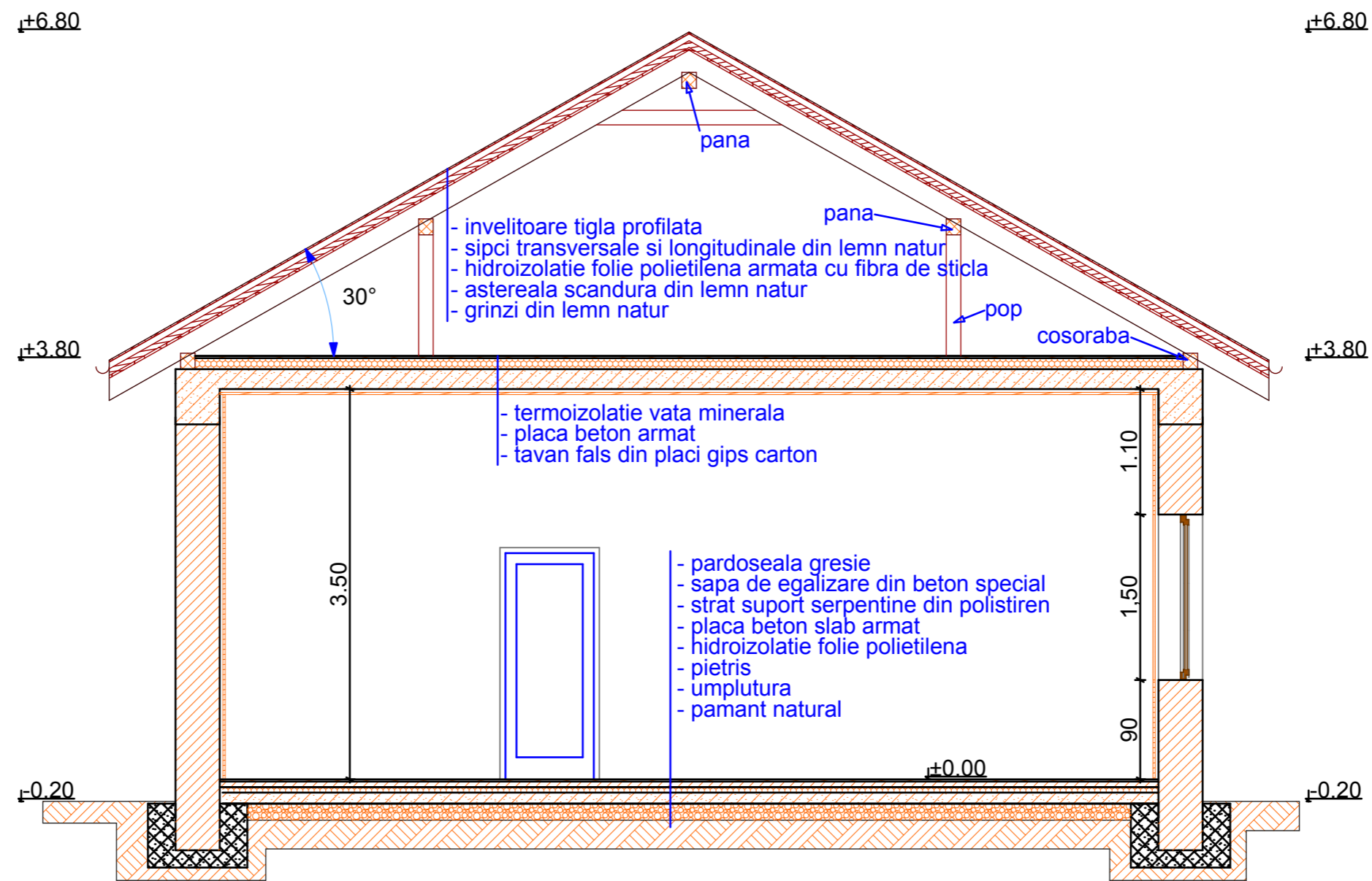
PROPUS - SECTIUNE B-B
